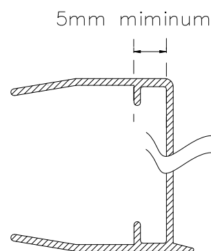
Figure 2 – Profilé de finition type dans le cas d'une prise en feuillure du vitrage organique multiparois sur 3 côtés (1 petit côté libre)
