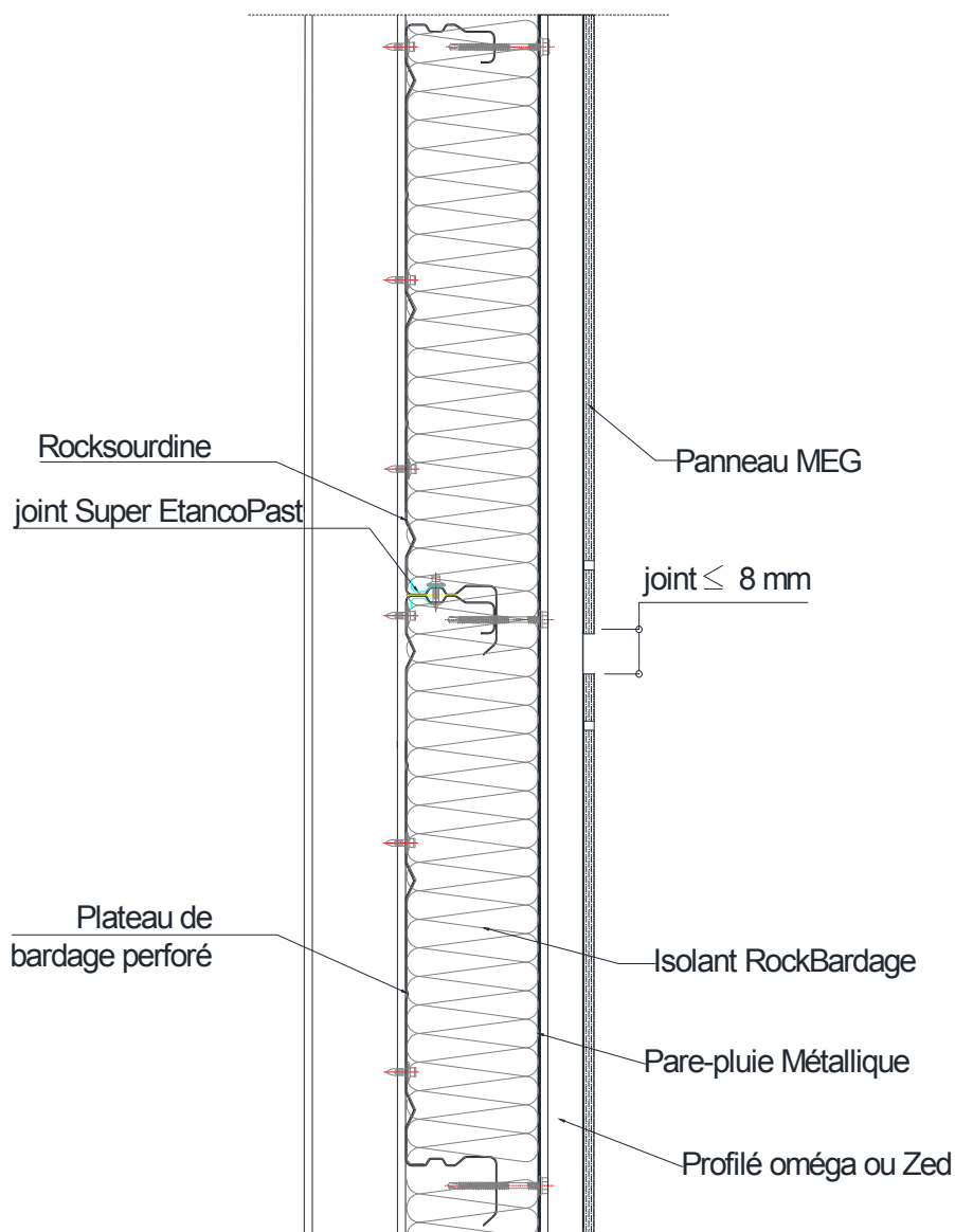
Figure 7 – Coupe verticale avec Rocksourline sur plateau perforé et joint super EtancoPast
