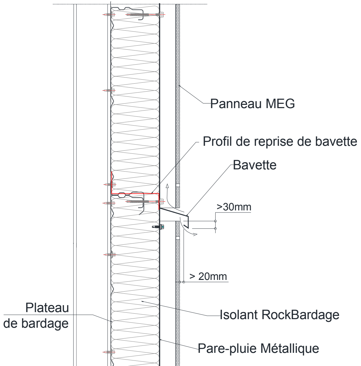
Figure 13 – Fractionnement de la lame d'air
