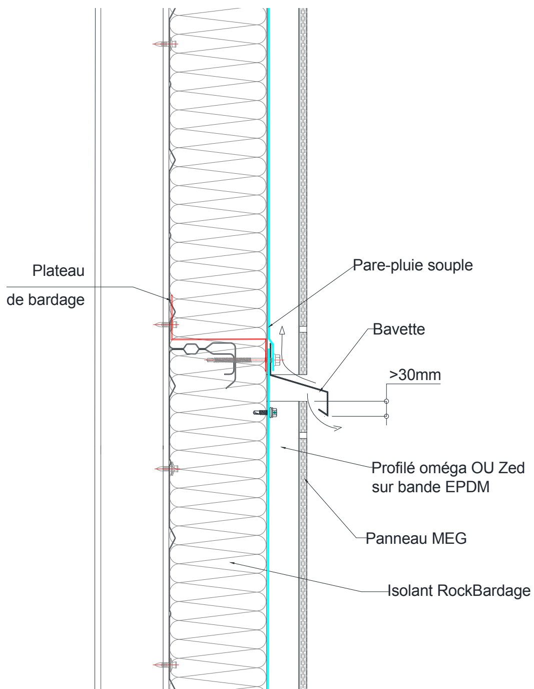
Figure 22 – Recouplement du pare pluie souple tous les 6m
