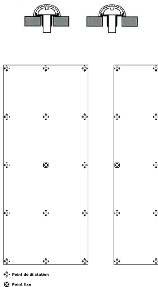
Figure 4 - Traitement des joints entre panneaux
