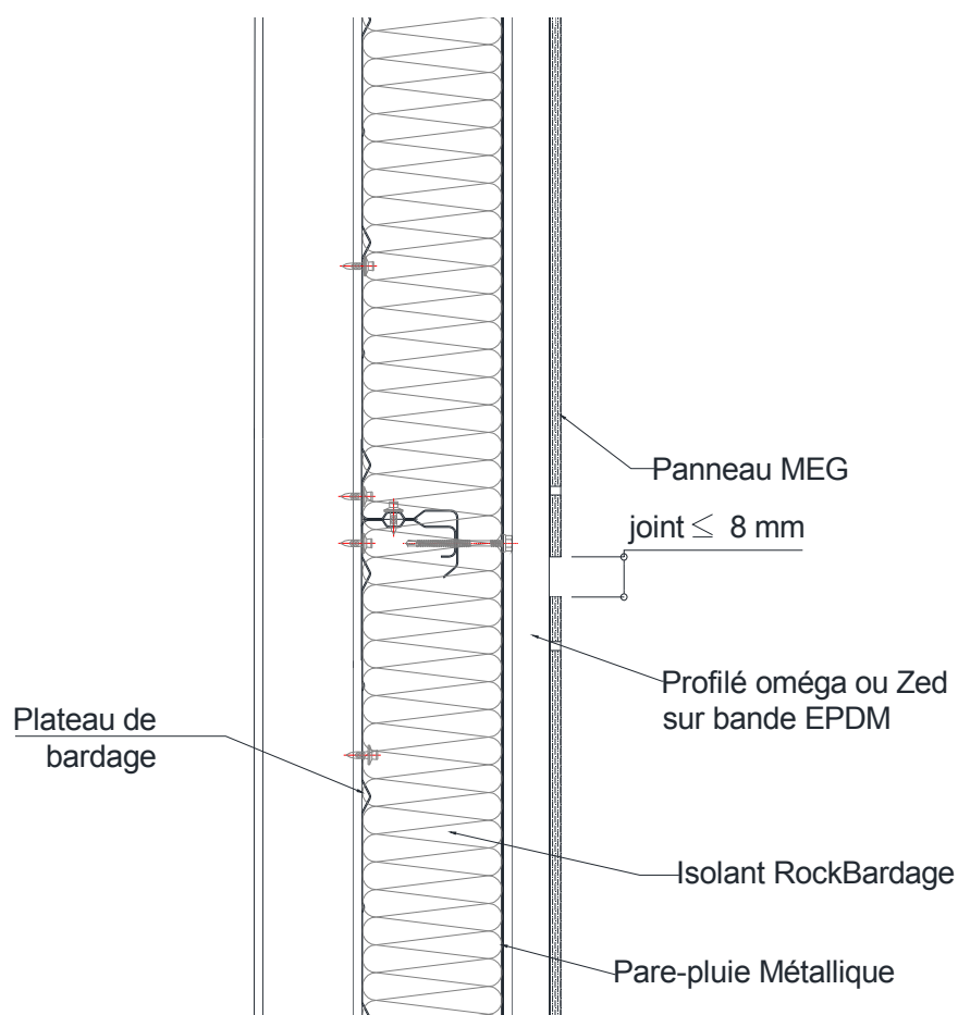
Figure 5 – Coupe verticale avec pare-pluie métallique
