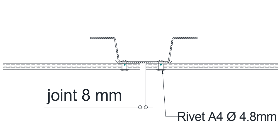
Figure 1.1 – Traitement du joint vertical entre panneaux
