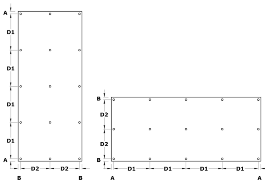
Figure 3.1 - Trois rangées de fixations
