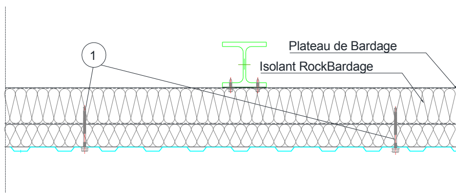
Figure 2 – Etapes de pose pare pluie / ossature / Panneaux
