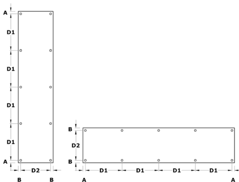
Figure 3.2 - Deux rangées de fixations
