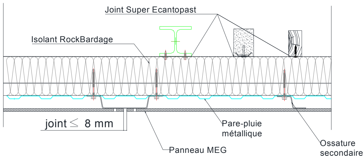
Figure 8 – Coupe horizontale avec pare-pluie métallique
