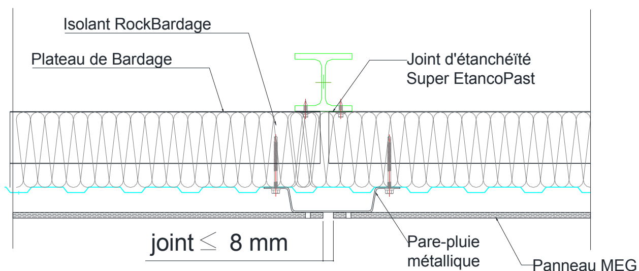
Figure 10 - Aboutage des plateaux
